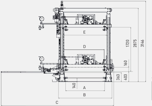
Movable machine configuration, with sliding strapping bayonet Konfigurácia pohyblivého stroja, s výsuvným páskovacím bajonetom
