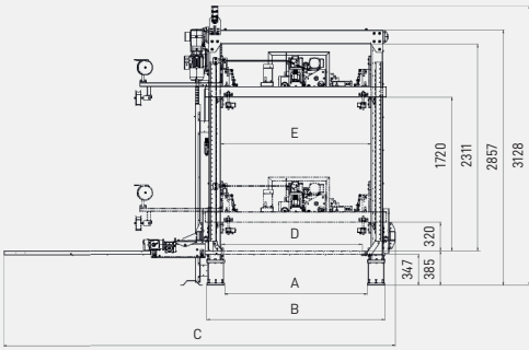
Configuration with sliding strapping bayonet Konfigurácia s výsuvným páskovacím bajonetom
